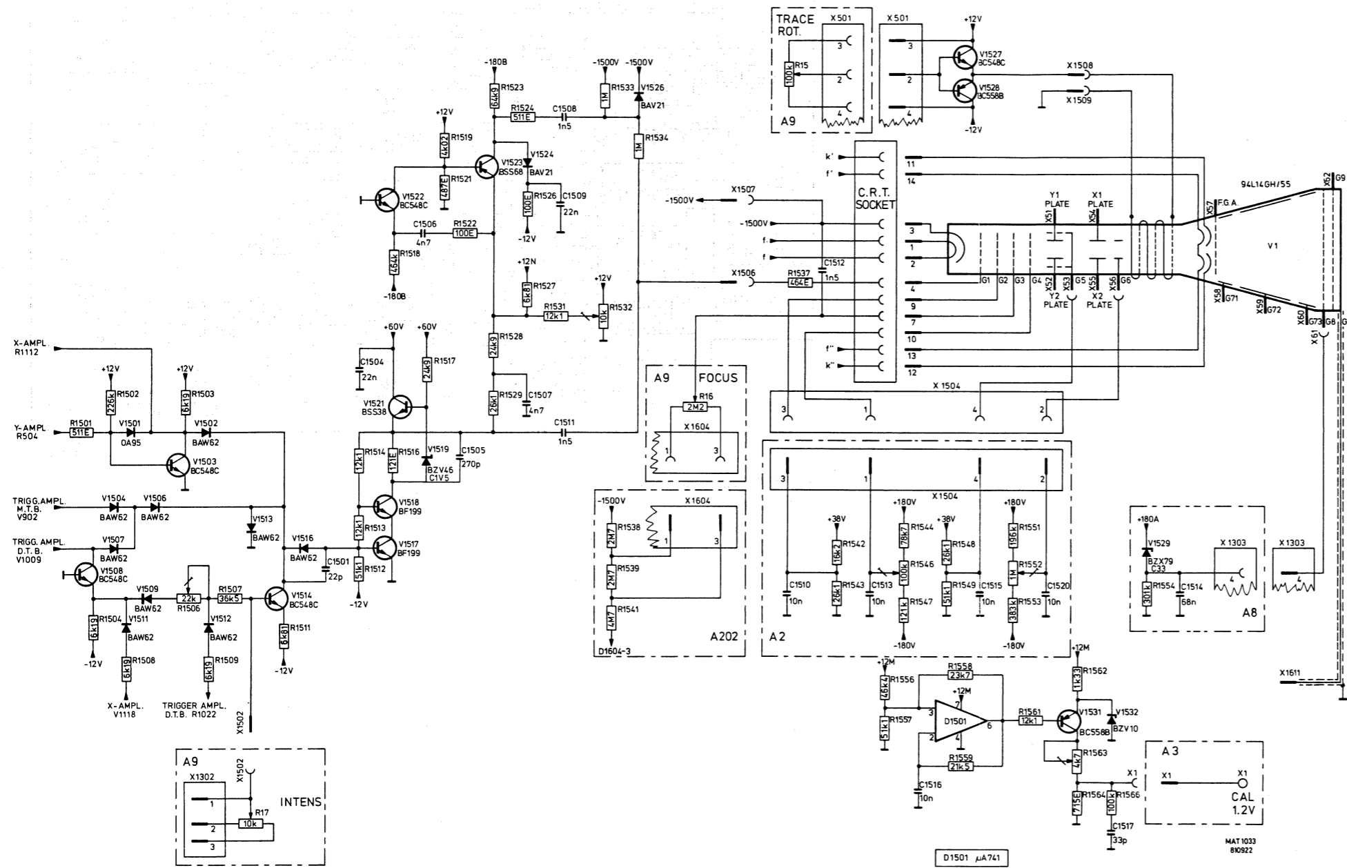
Fig. 8.8. Z-Amplifier
